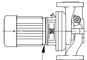
Fig. 25 Drain hole
